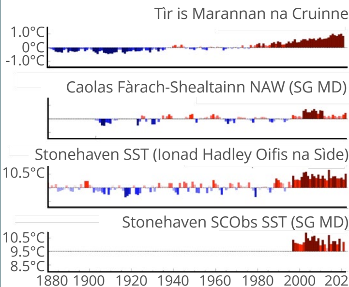
Ìomhaigh 1: Grafaichean a' sealltainn atharraichean ann an teothachd nan cuantan eadar 1880 is 2020 ann an diofar àiteachan.
